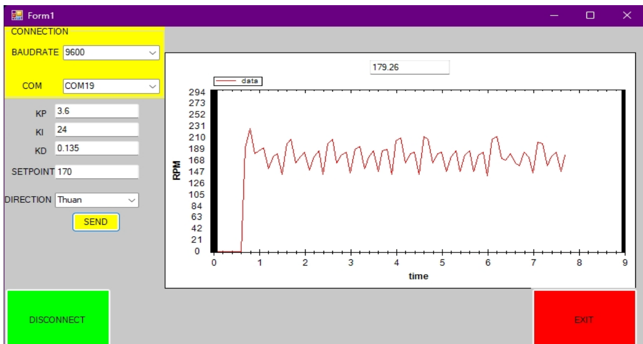
Hình 21: Đồ thị đáp ứng với K_p , K_i , K_d vừa tính được tại Setpoint = 170 RPM
