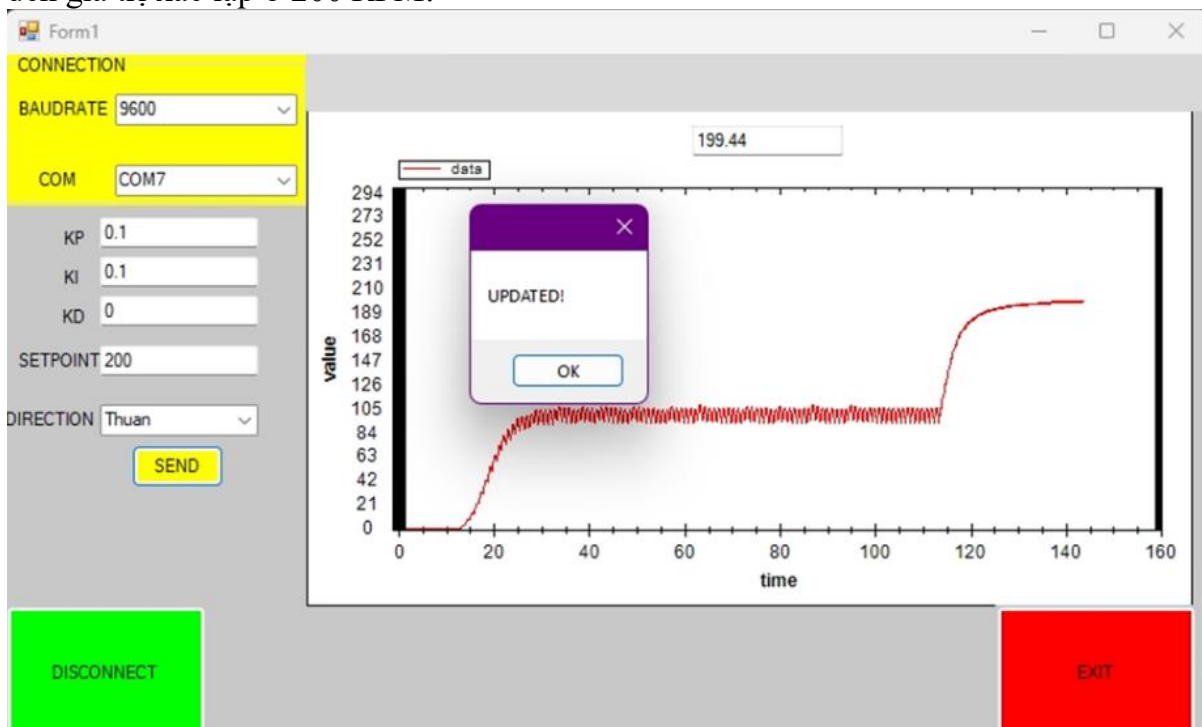
Hình 17: Setpoint=200 RPM
