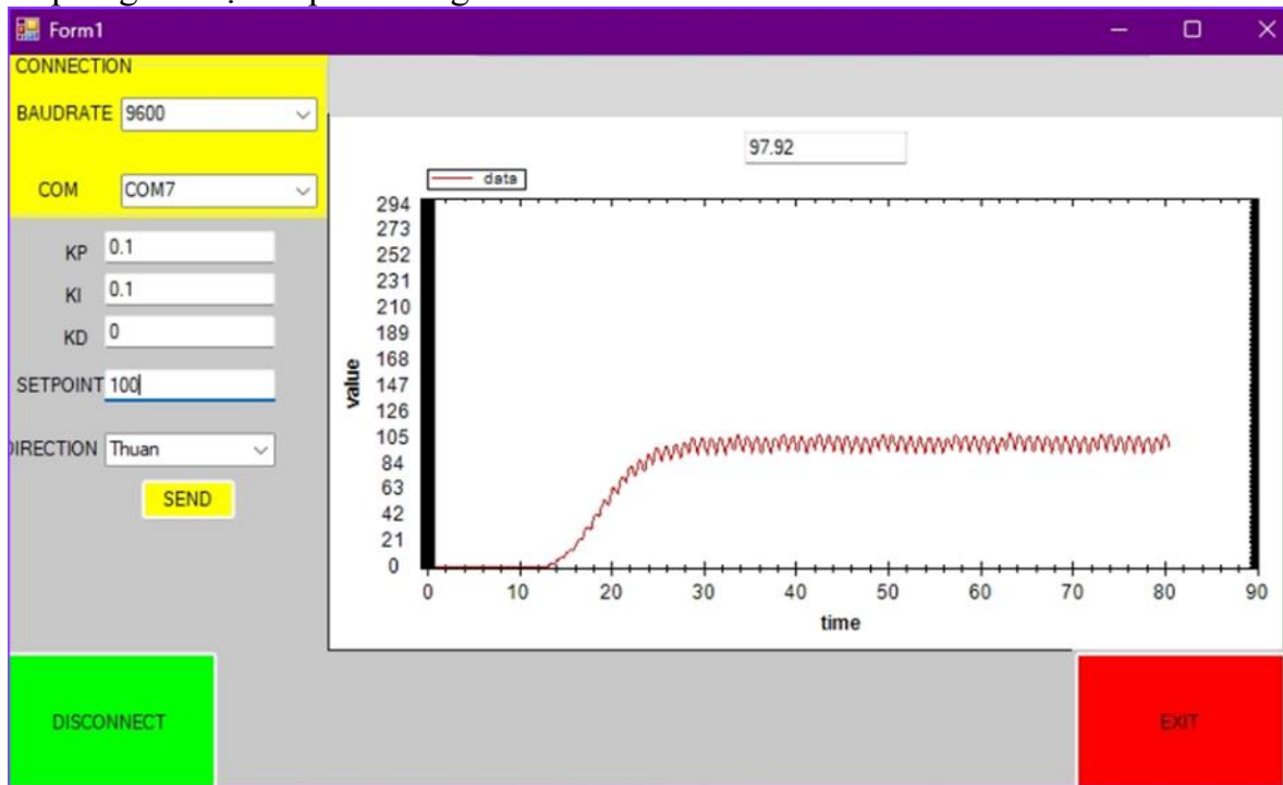
Hình 16: Setpoint=100 RPM
